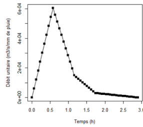
Hydrogramme unitaire
