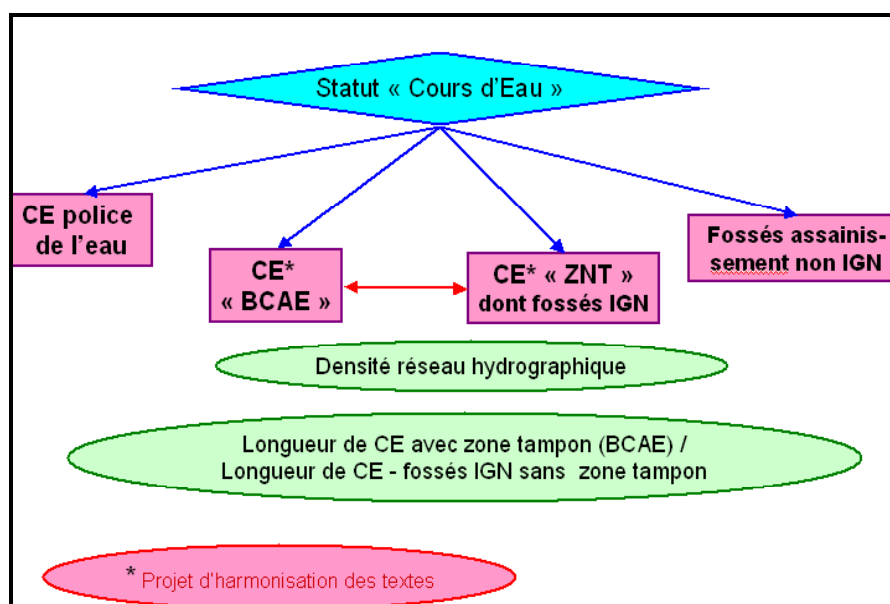
Figure 11 : différenciation des écoulements hydrauliques selon leurs statuts réglementaires
