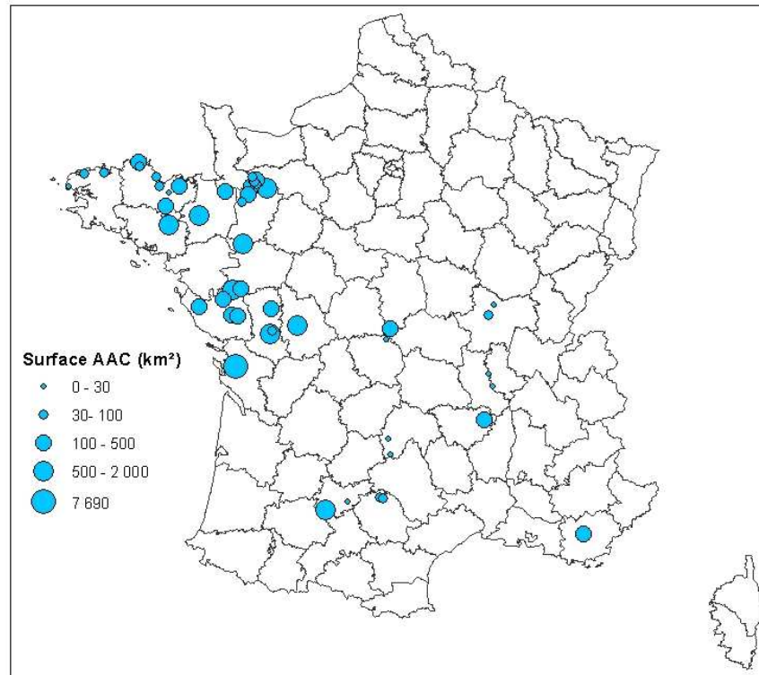
Figure 1 : localisation des captages Grenelle métropolitains en eaux de surface (données Agences de l'Eau)
