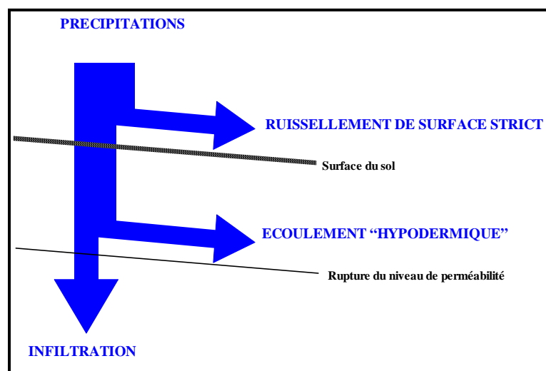
Figure 3: les voies de transferts hydriques dans le sol (CORPEN, 1999)
