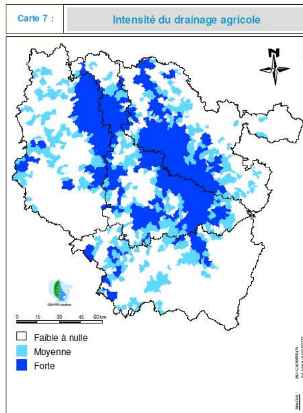
Figure 8 : exemple d'intensité de drainage agricole à l'échelle régionale (GRAPPE Lorraine, 2006).
