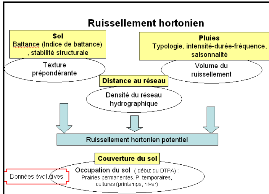
Figure 5 : facteurs générant le ruissellement hortonien
