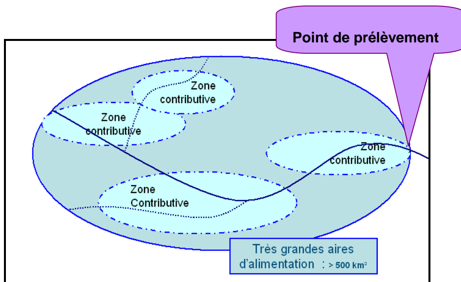
Figure 13: priorisation des zones de diagnostic dans le cas de très grandes aires
