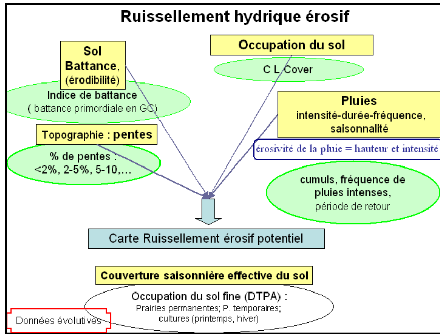
Figure 9 : paramètres retenus pour évaluer l'érosion hydrique
