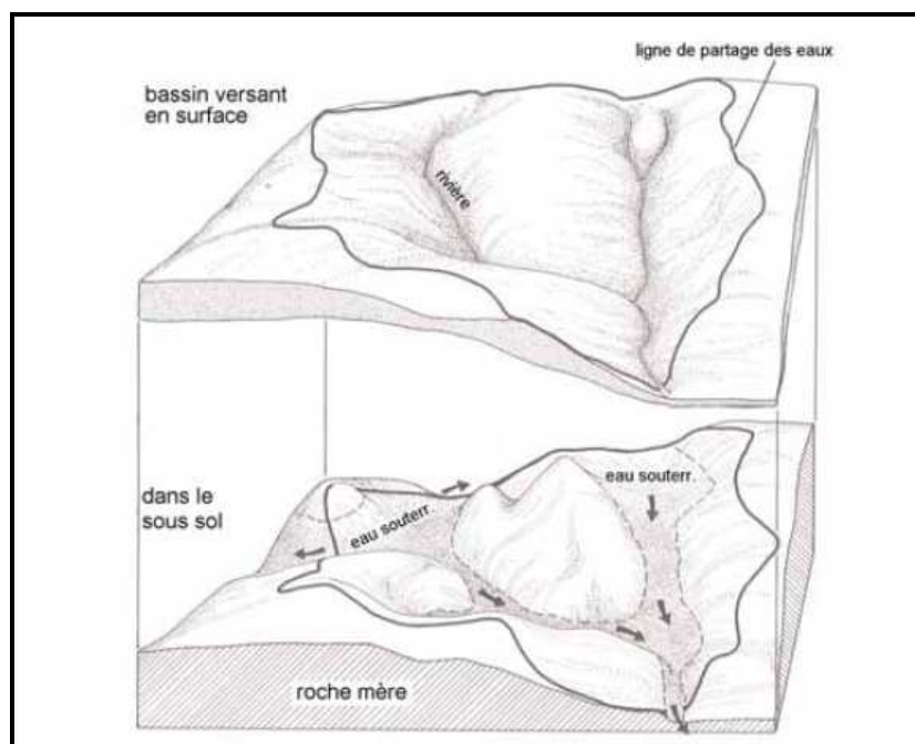
Figure 2 : notion de bassin versant (CORPEN, 2007, d'après Andréassian, 2005)
