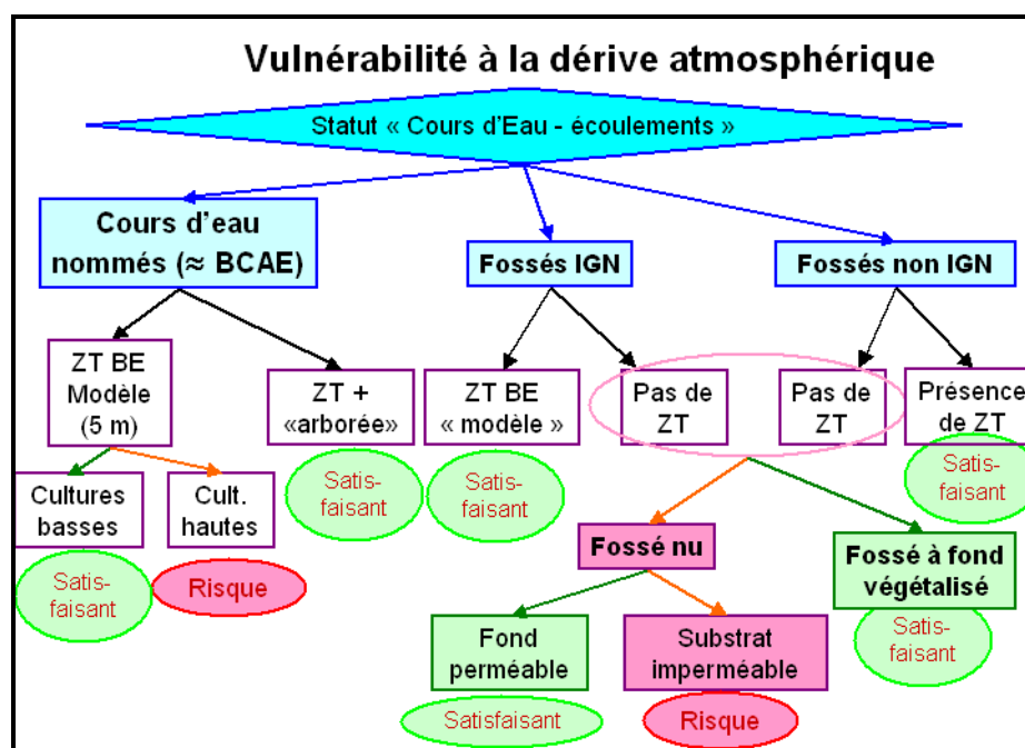
Figure 12 : Efficacité de la protection contre la dérive des embruns Proposition d'arbre de décision
