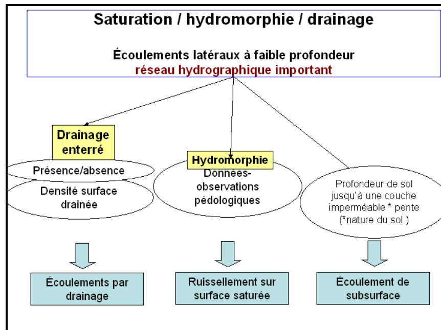
Figure 6 : partition des écoulements latéraux à faibles profondeurs
